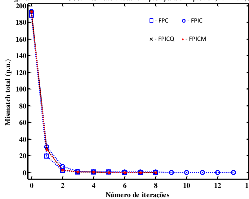
Figura 22 – IEEE-300: Mismatch total em p.u. para \lambda=1 p.u. e 1,472 \cdot R/1,0 \cdot X .
